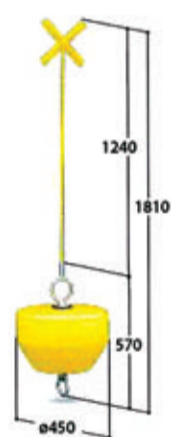
UMB-30 Markerings/bade bøye Volum 30 liter Art. no 3267054 Vekt 8,0 kg
